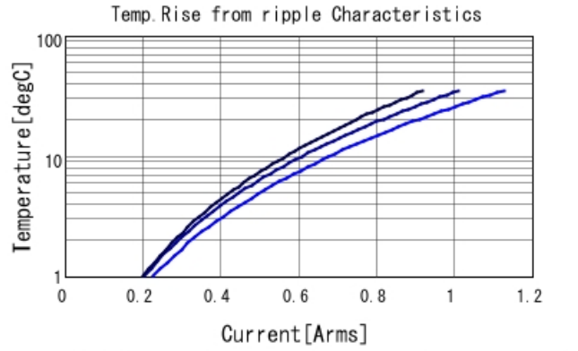
GRM1555C1H300JA01 Temp. rise — 500MHz — 700I
