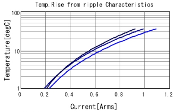
GRM1555C1H220JA01 Temp. rise — 500MHz — 700I
