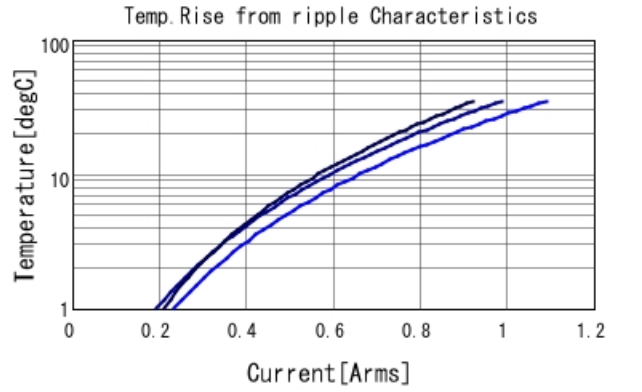
GRM1555C1H220GA01 Temp. rise — 500MHz — 700V
