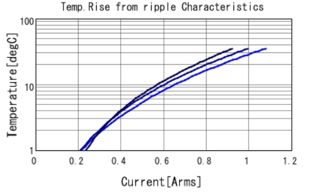
GRM1555C1H200JA01 Temp. rise — 500MHz — 700I
