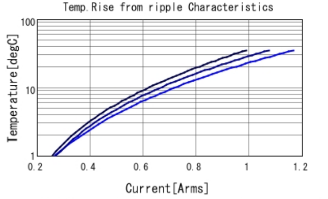
GRM1555C1H150JA01 Temp. rise — 500MHz — 700I
