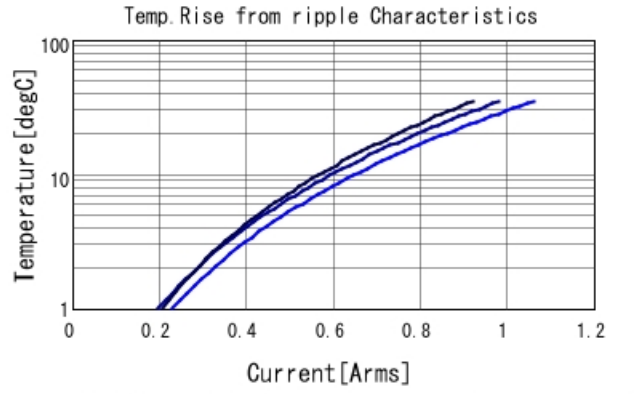
GRM1555C1H120JA01 Temp. rise — 500MHz — 700I
