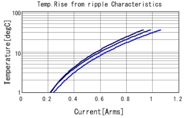
GRM1555C1H110JA01 Temp. rise — 500MHz — 700I
